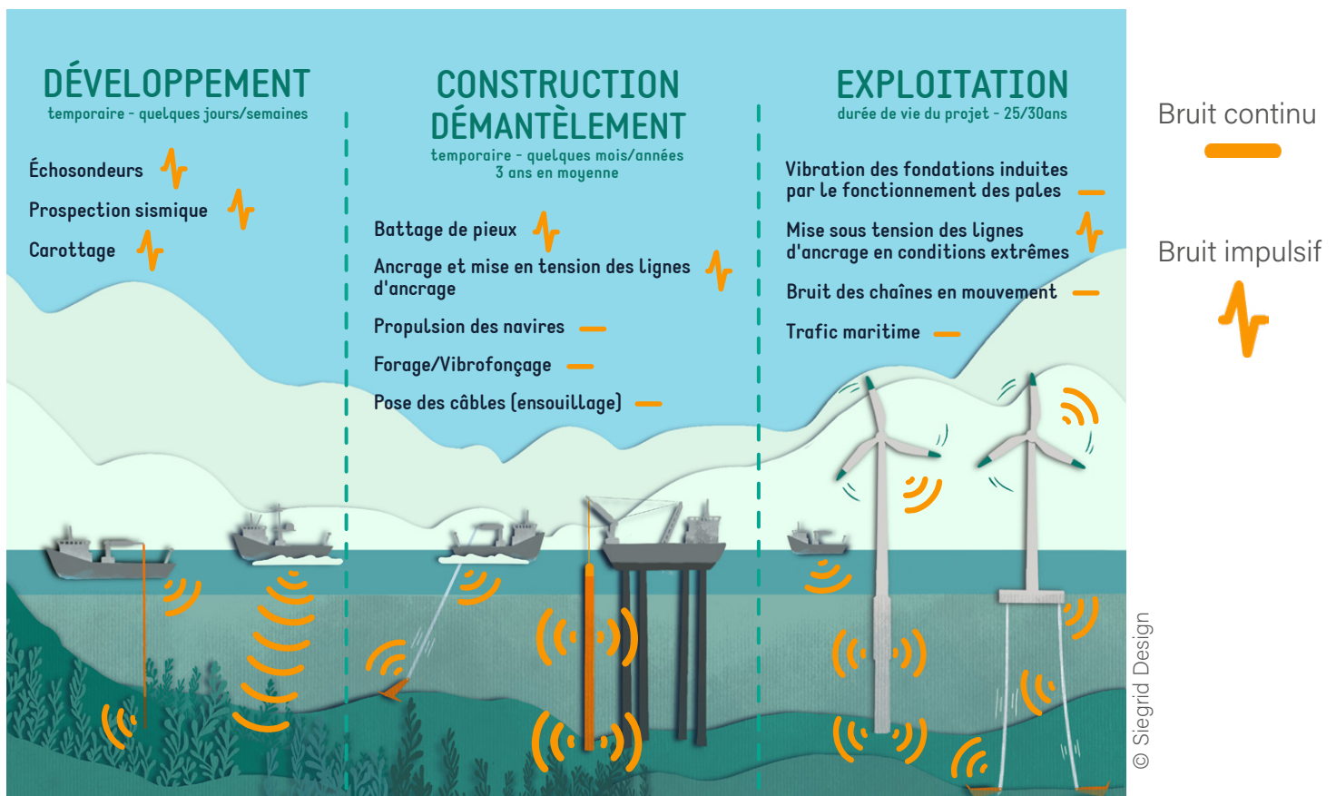
Fig. 4 Synthèse des principales sources d'émissions sonores associées à toutes les phases du cycle de vie d'un parc éolien en mer (allant de la prospection au démantèlement) en fonction du type d'infrastructure (posé ou flottant) et d'activité (prospection, trafic maritime, etc.). Les types de sons émis sont indiqués par les lignes orange. L'énergie acoustique des différentes sources d'émissions en fonction de la distance, du type de bruit, etc. n'est pas représentée ici (D'après Popper et al., 2022).
