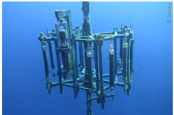
Dispositif avec coupons de polyéthylène haute densité (PEHD) et de polytéréphtalate d'éthylène (PET) pour le suivi de la biocolonisation des ancrages et câbles électriques et la quantification de l'hydrodynamisme
